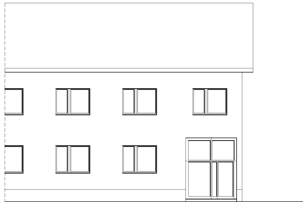
ELEWACJA ZACHODNIA
