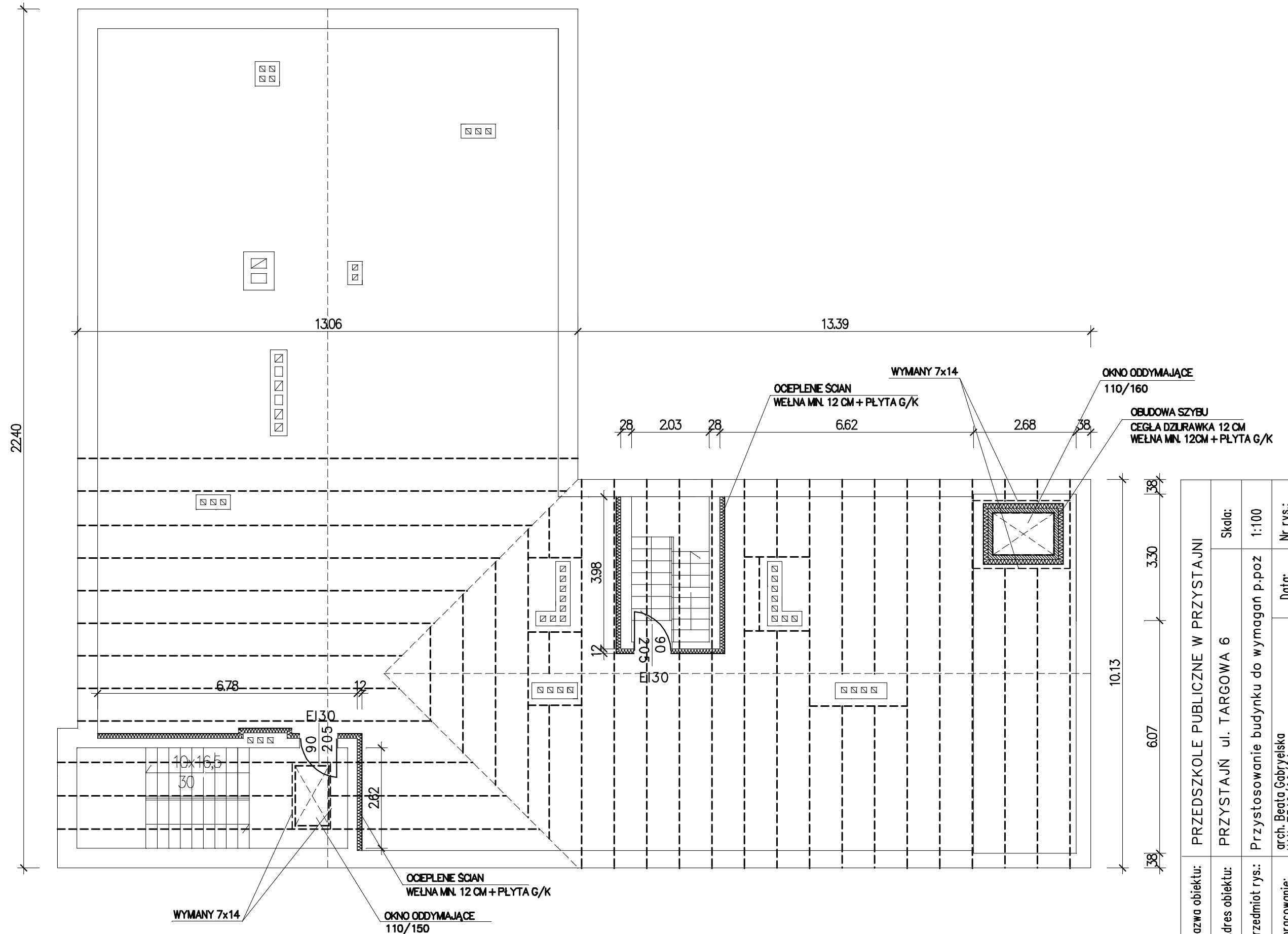
RZUT PODDASZA - PROJEKTOWANE ZMIANY
