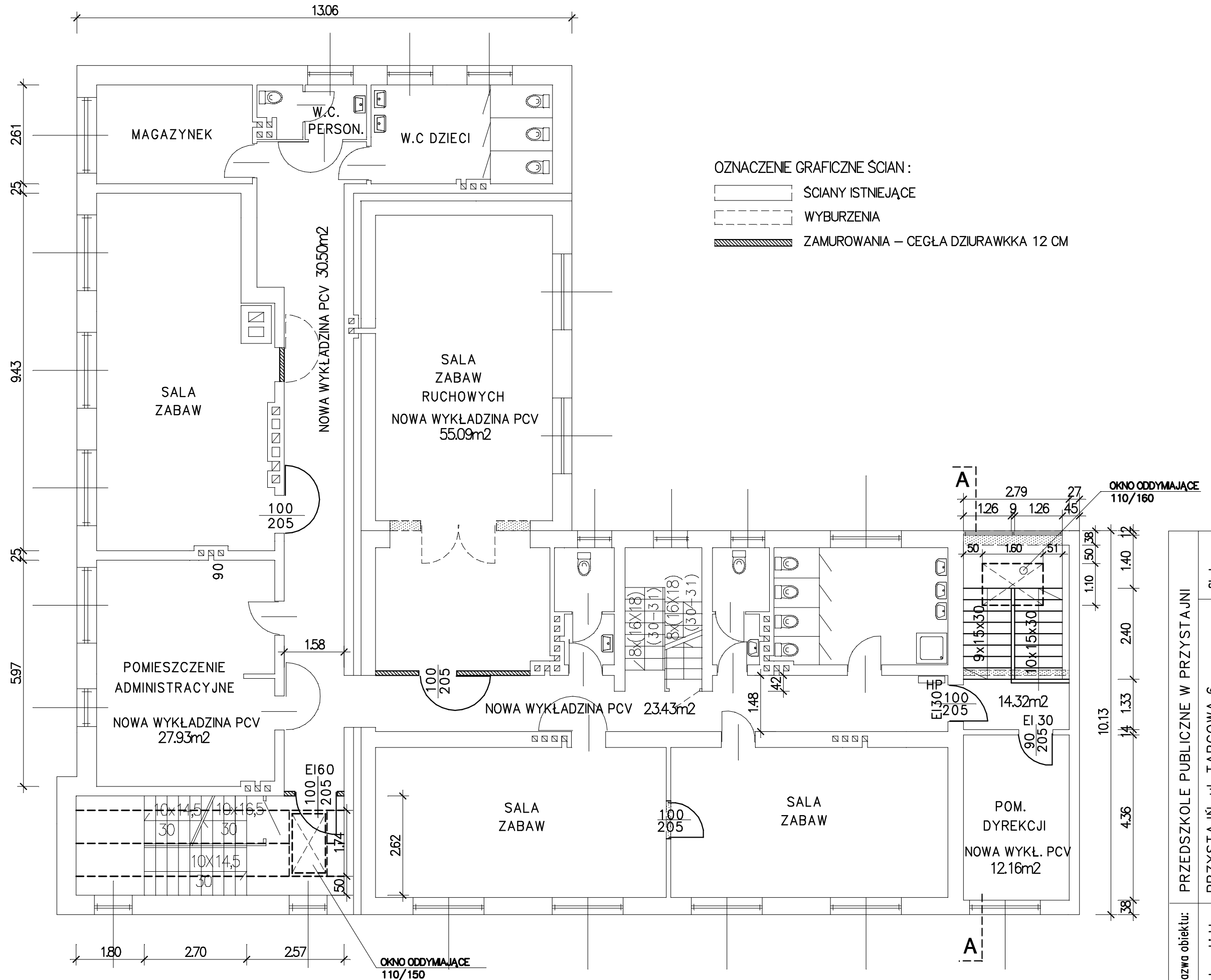
RZUT PIĘTRA - PROJEKTOWANE ZMIANY
