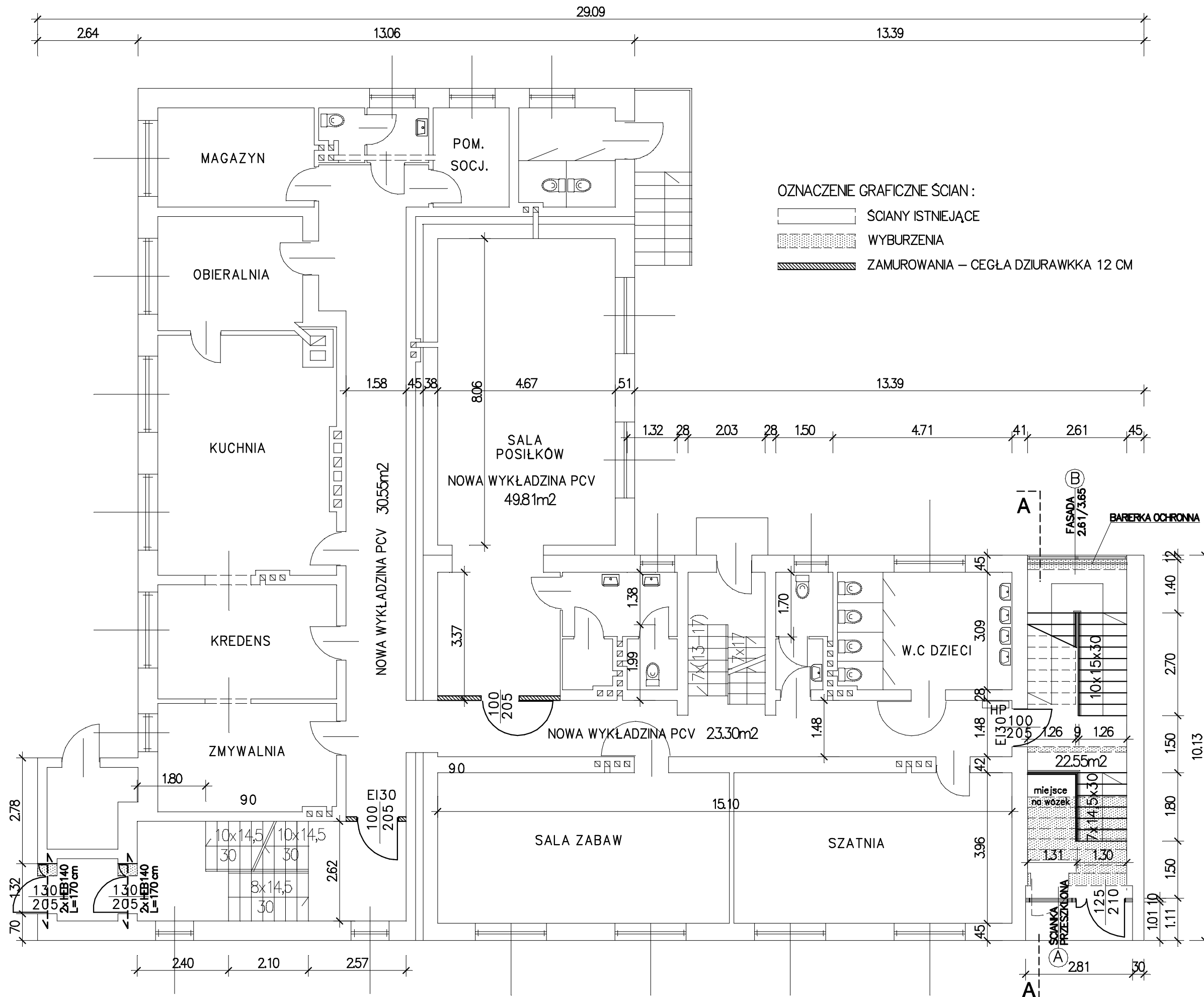
RZUT PRZYZIEMIA - PROJEKTOWANE ZMIANY
