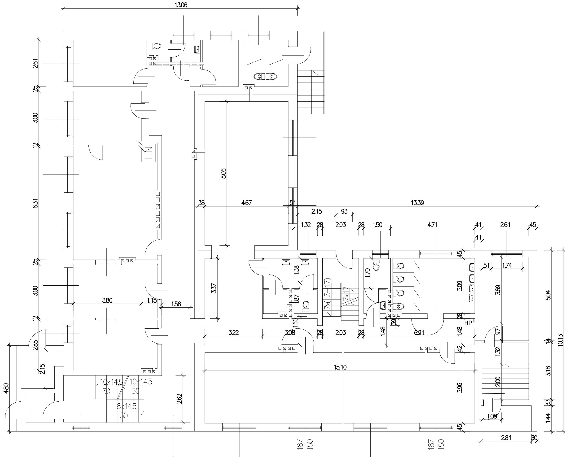
RZUT PRZYZIEMIA - STAN ISTNIEJĄCY
