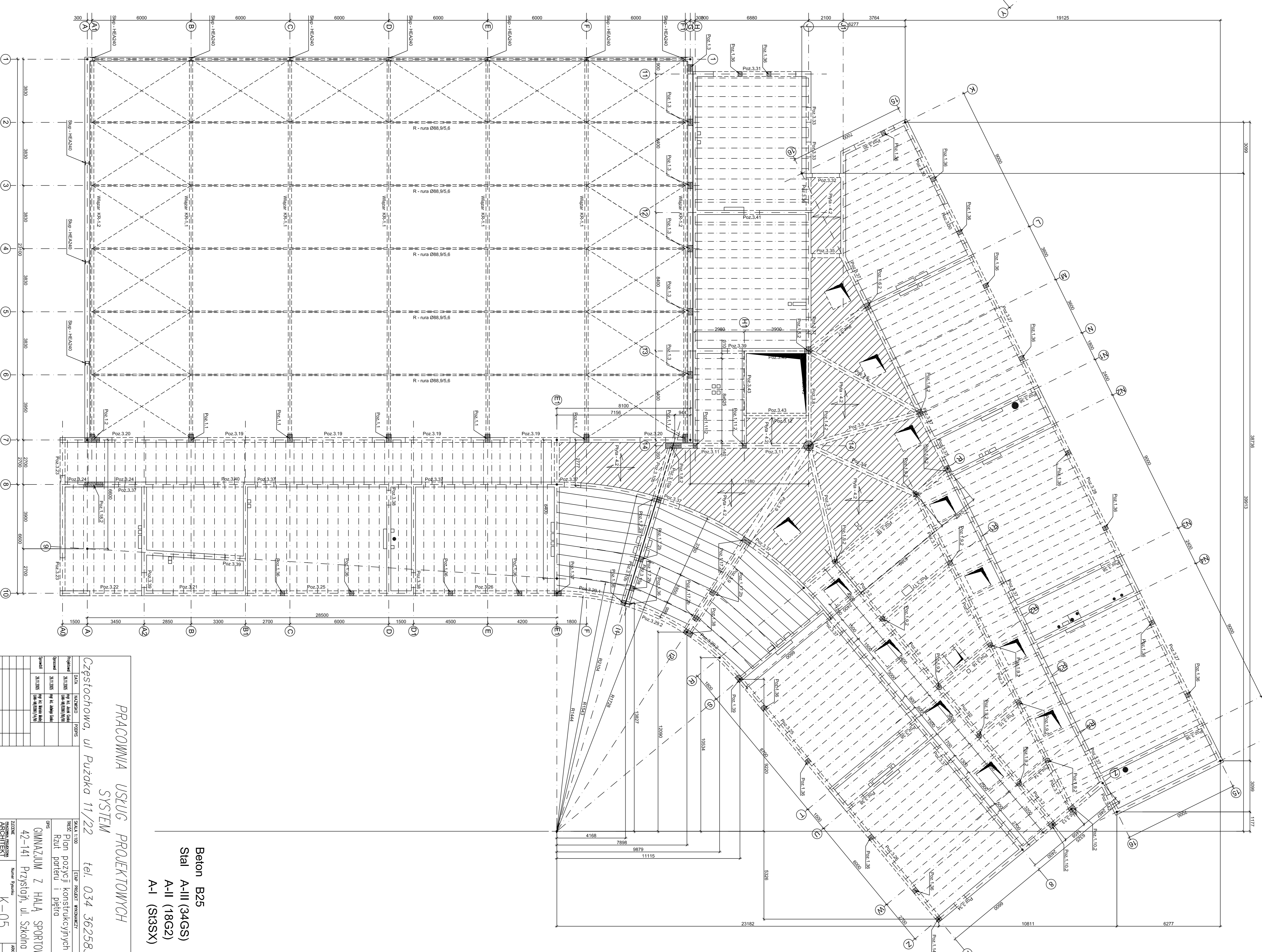
PLAN ELEMENTÓW KONSTRUKCYJNYCH - PIĘTRO 1:100
