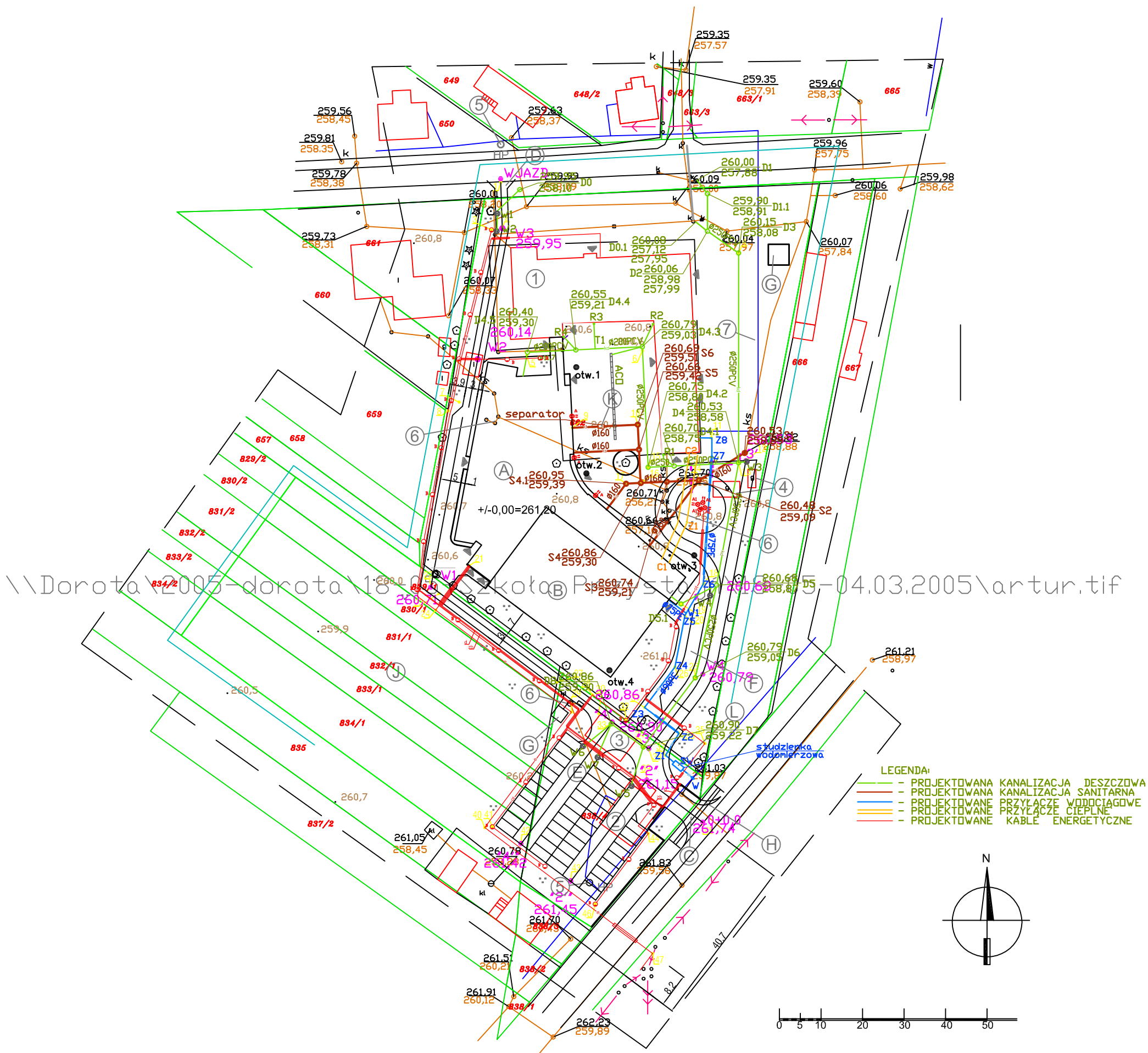
PLAN ZAGOSPODAROWANIA TERENU 1:1000
